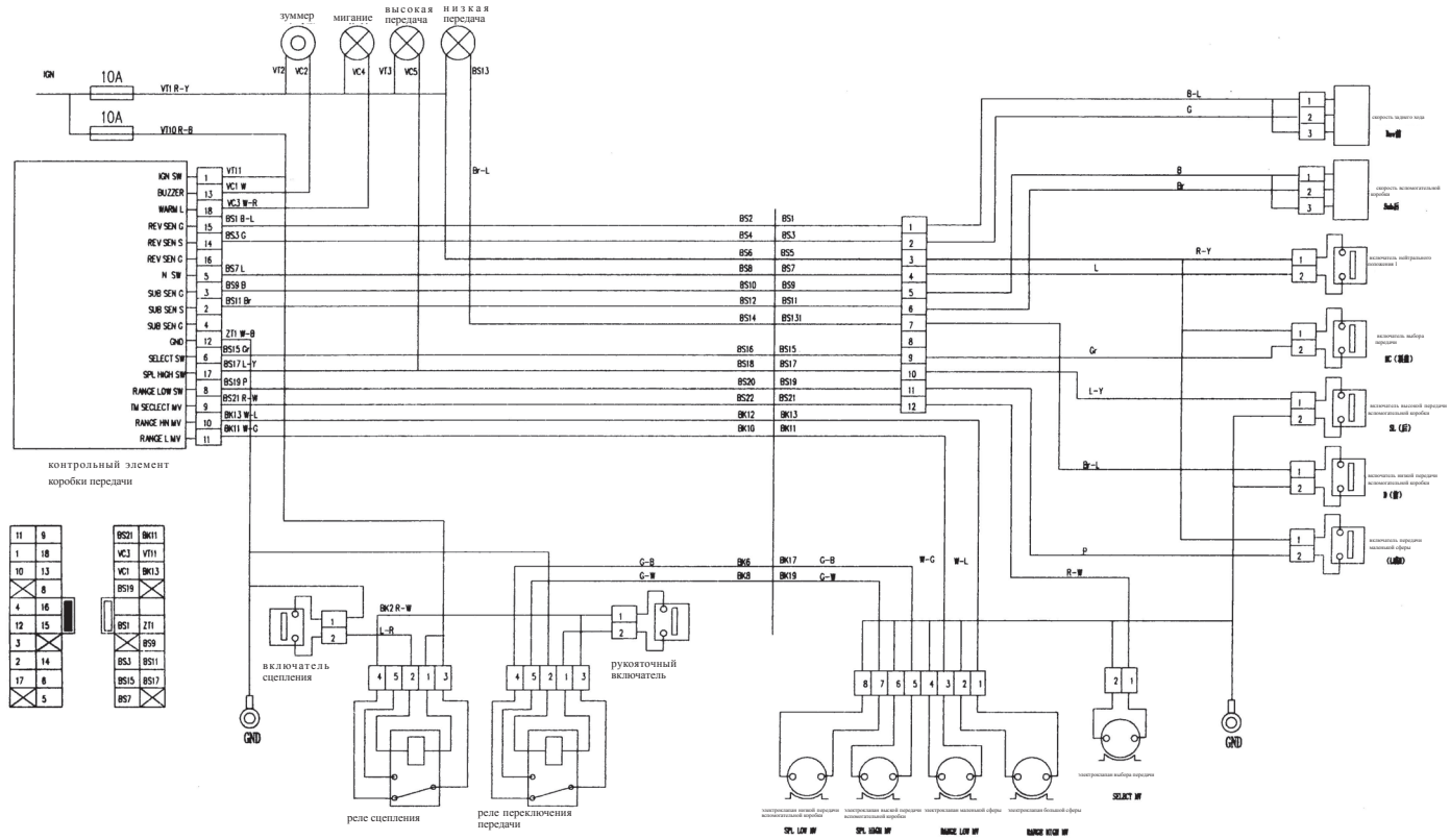
принципиальная схема коробки передач с 12 передачами большой шестерни
